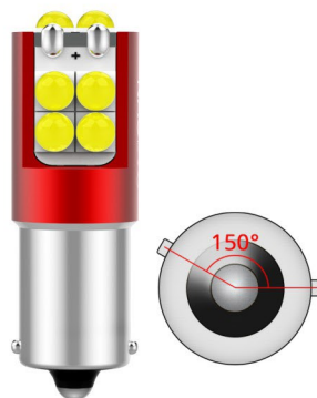
BAY9S
